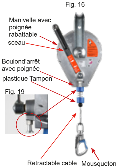
Figure 16 / 19 montre: L'antichute à rappel automatique IKAR avec la position de la manivelle en fonctionnement sur l'antichute à rappel automatique
